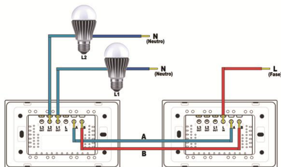
VL-C302S-81, VL-C302S-82
