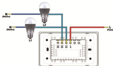
VL-C302-81, VL-C302-82
