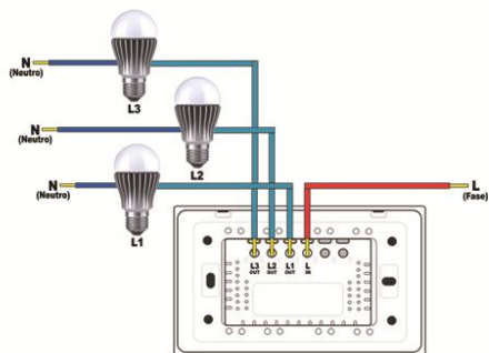
VL-C303-81, VL-C303-82
