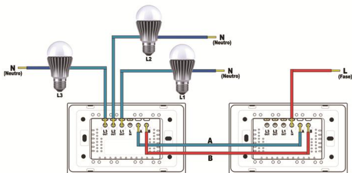
VL-C303S-81, VL-C303S-82
