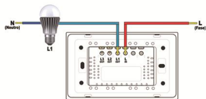
VL-C301-81, VL-C301-82
